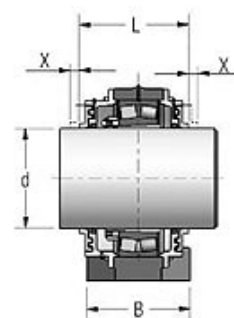
Execução Passante
